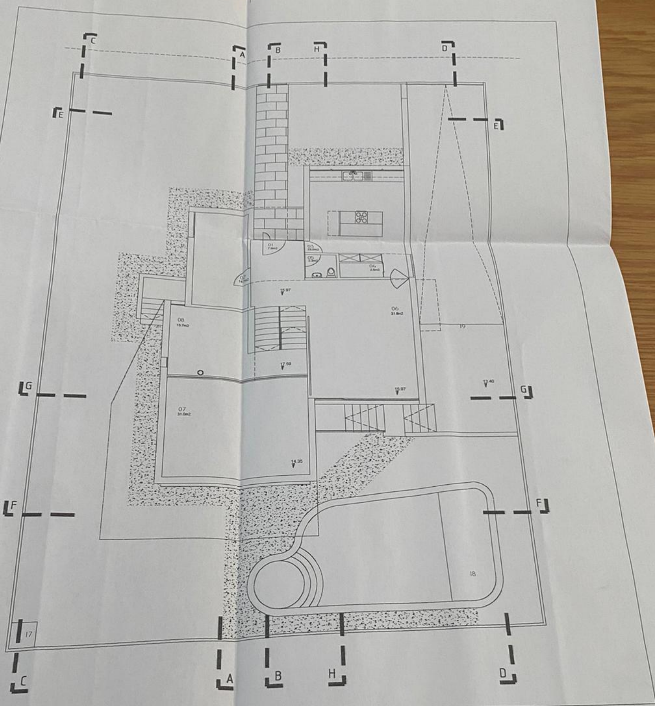
PLANTA DO RÉS DO CHÃO
