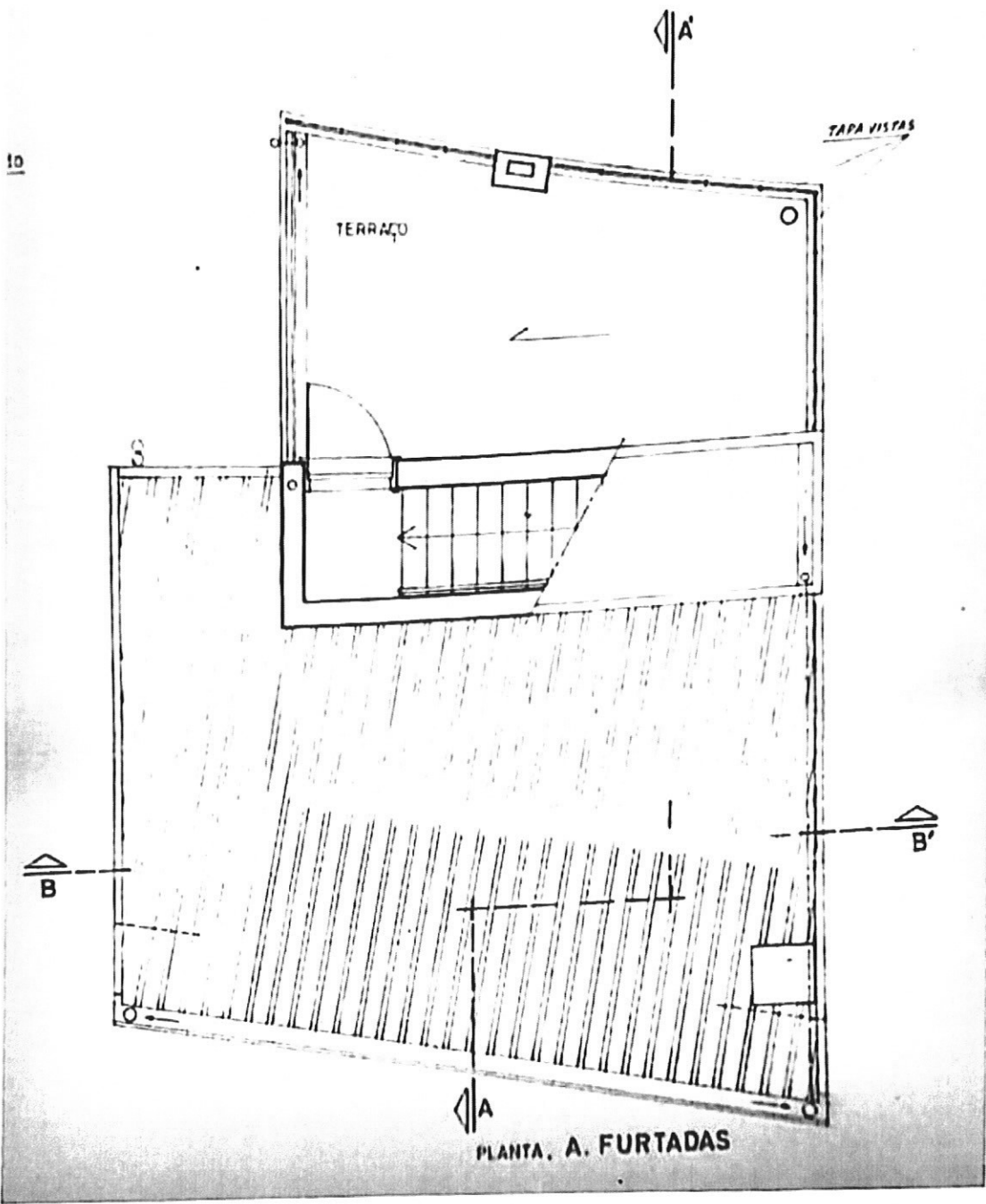
PLANTA DA COBERTURA (ESC: 1/100)
