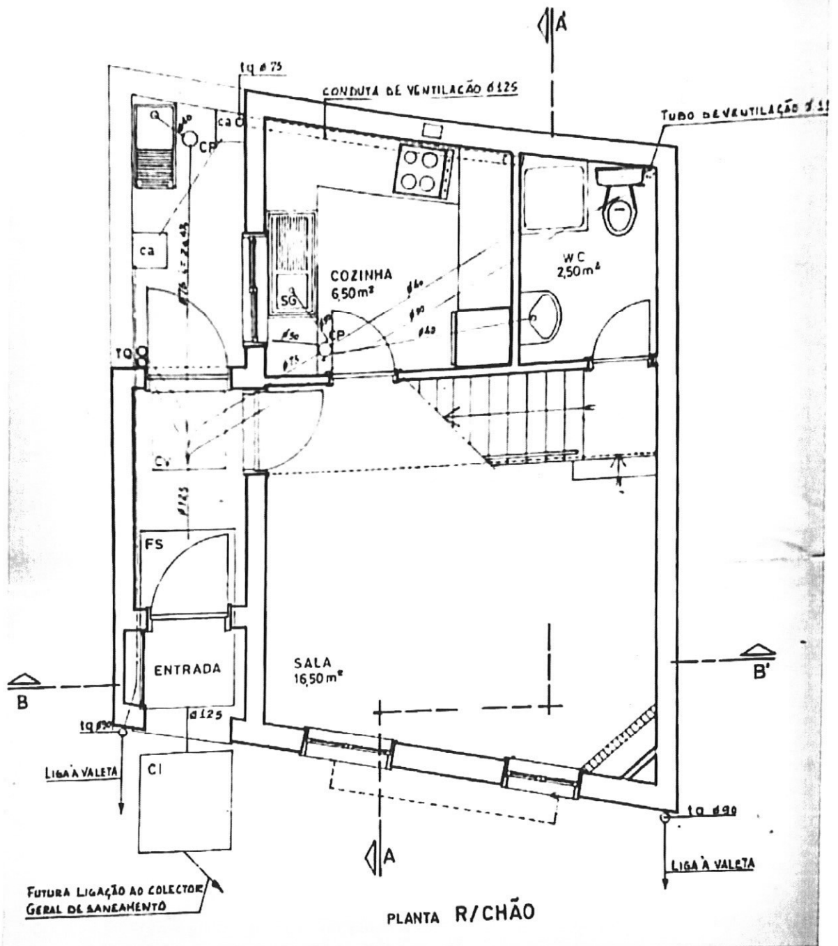
PLANTA DO RÉS-DO-CHÃO (ESC: 1/100)
