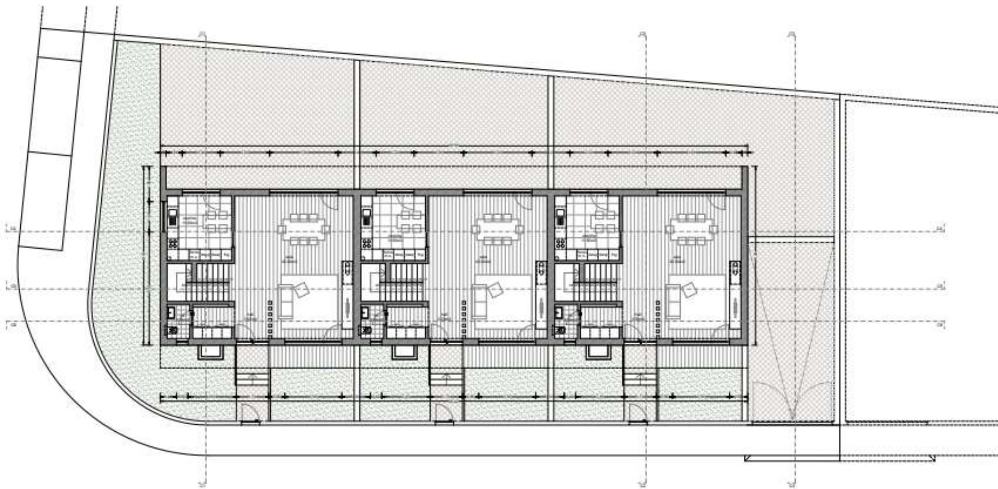
Rés-do-Chão 3 Moradias
