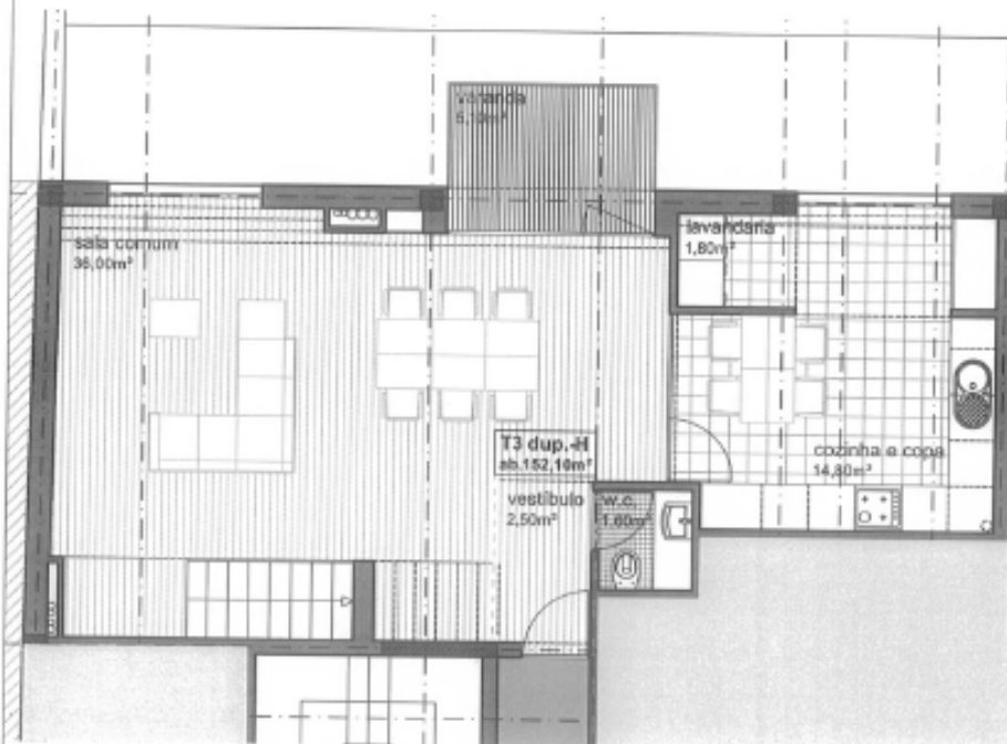
PLANTA DO APARTAMENTO_PISO 3
