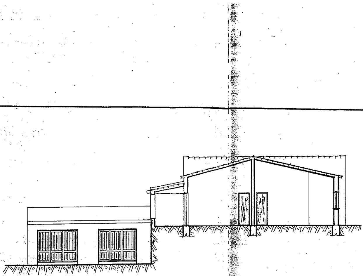
Corte A-B
