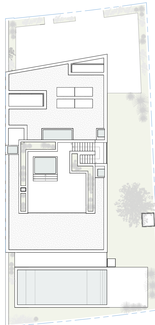
Planta de Cobertura | 1:200
