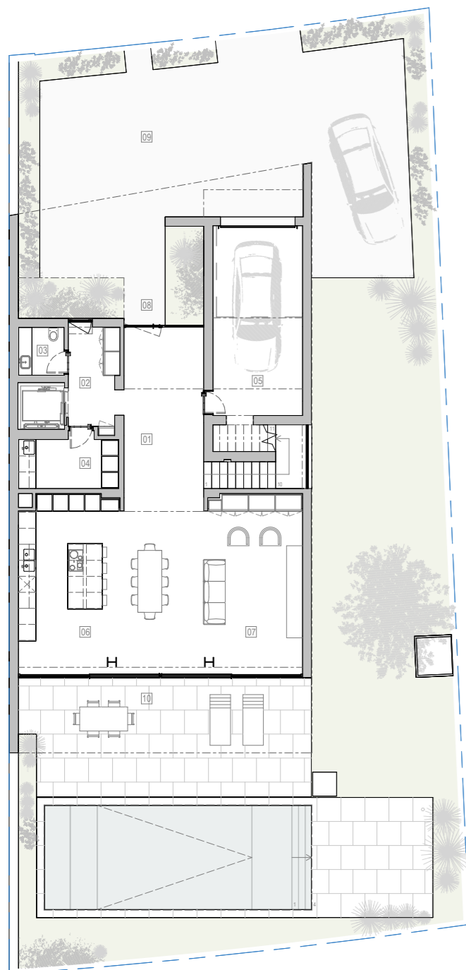
Planta do Piso 0 | 1:200
