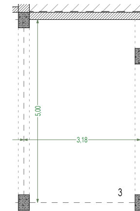
Lugar estacionamento _esc: 1/100
