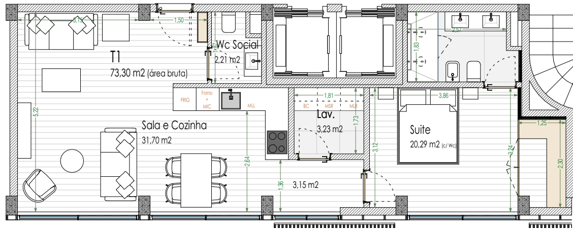
Planta Apartamento _esc: 1/100
