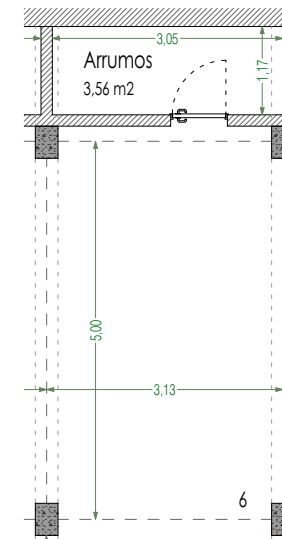
Lugar estacionamento _esc: 1/100
