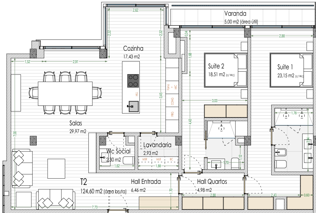
Planta Apartamento _ esc: 1/100
