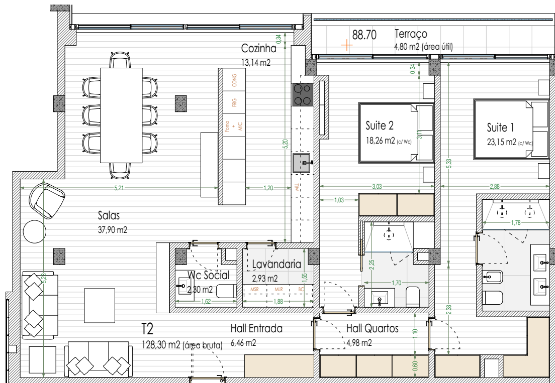
Planta Apartamento _esc: 1/100
