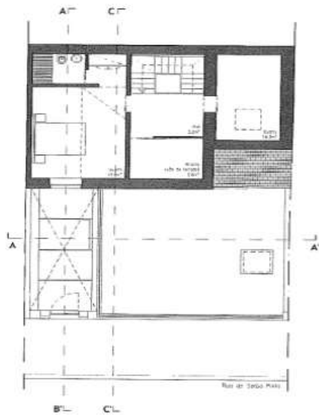
Planta do 1.º Piso
