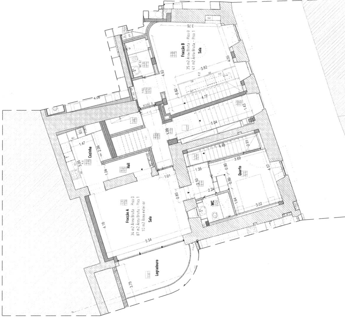
Planta da Habitação Piso 1
