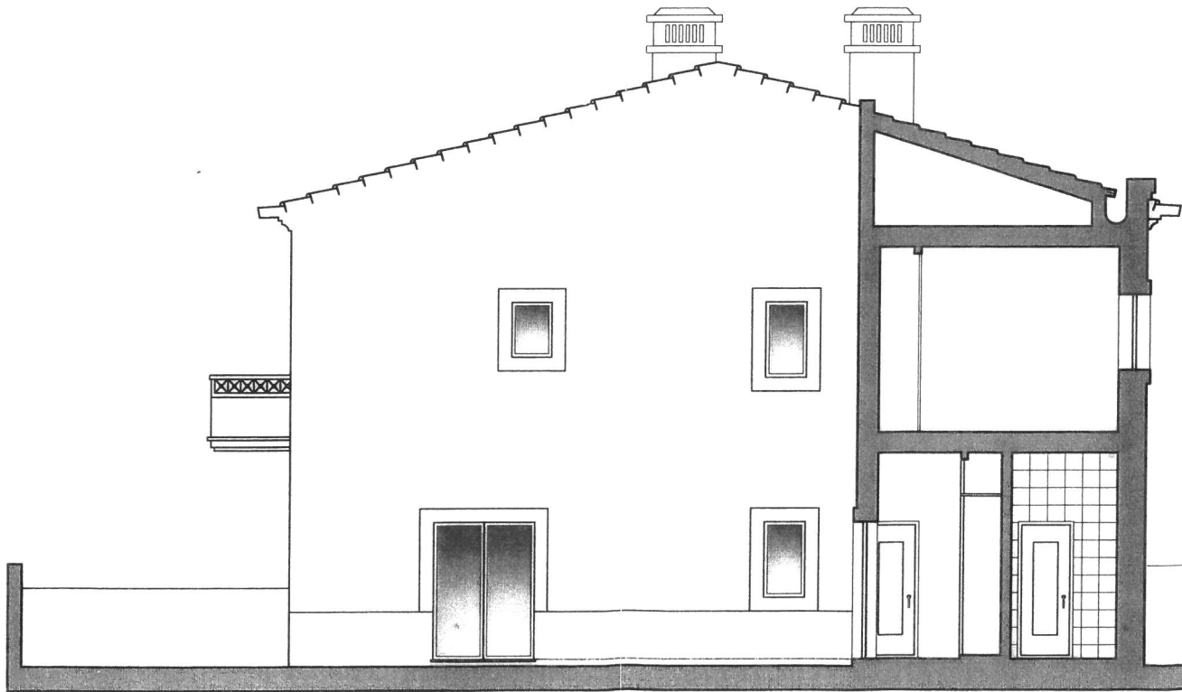
CORTE E/F
