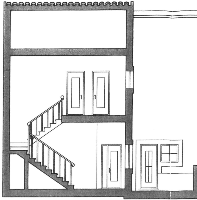
CORTE C/D
