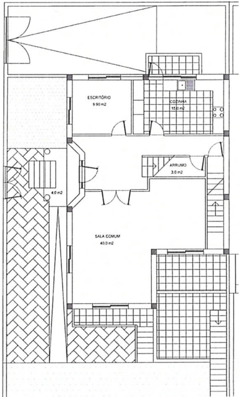
PLANTA DO RÉS-DO-CHÃO
