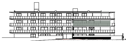
ALÇADO POSTERIOR
