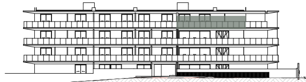
ALÇADO POSTERIOR
