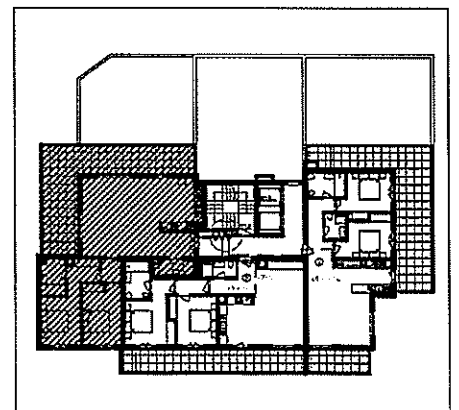
PISO 8
