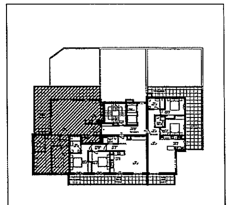
PISO 8
