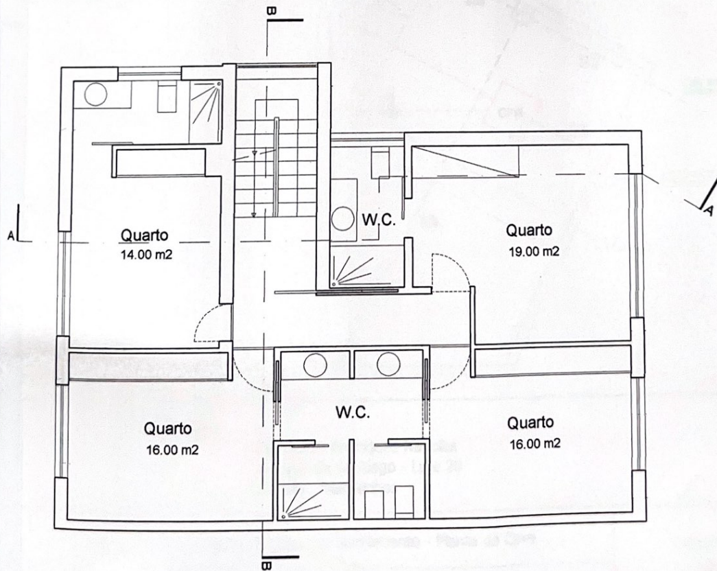
PLANTA DO ANDAR
