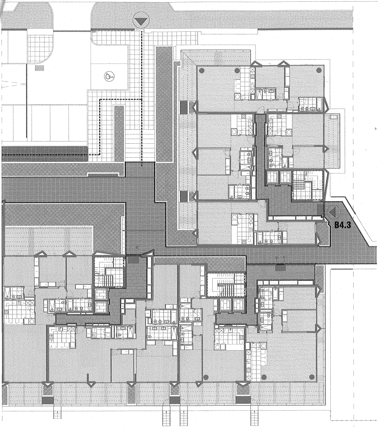
PLANTA PISO 1 ENTRADA - BLOCO 4 - Esc. 1:300
