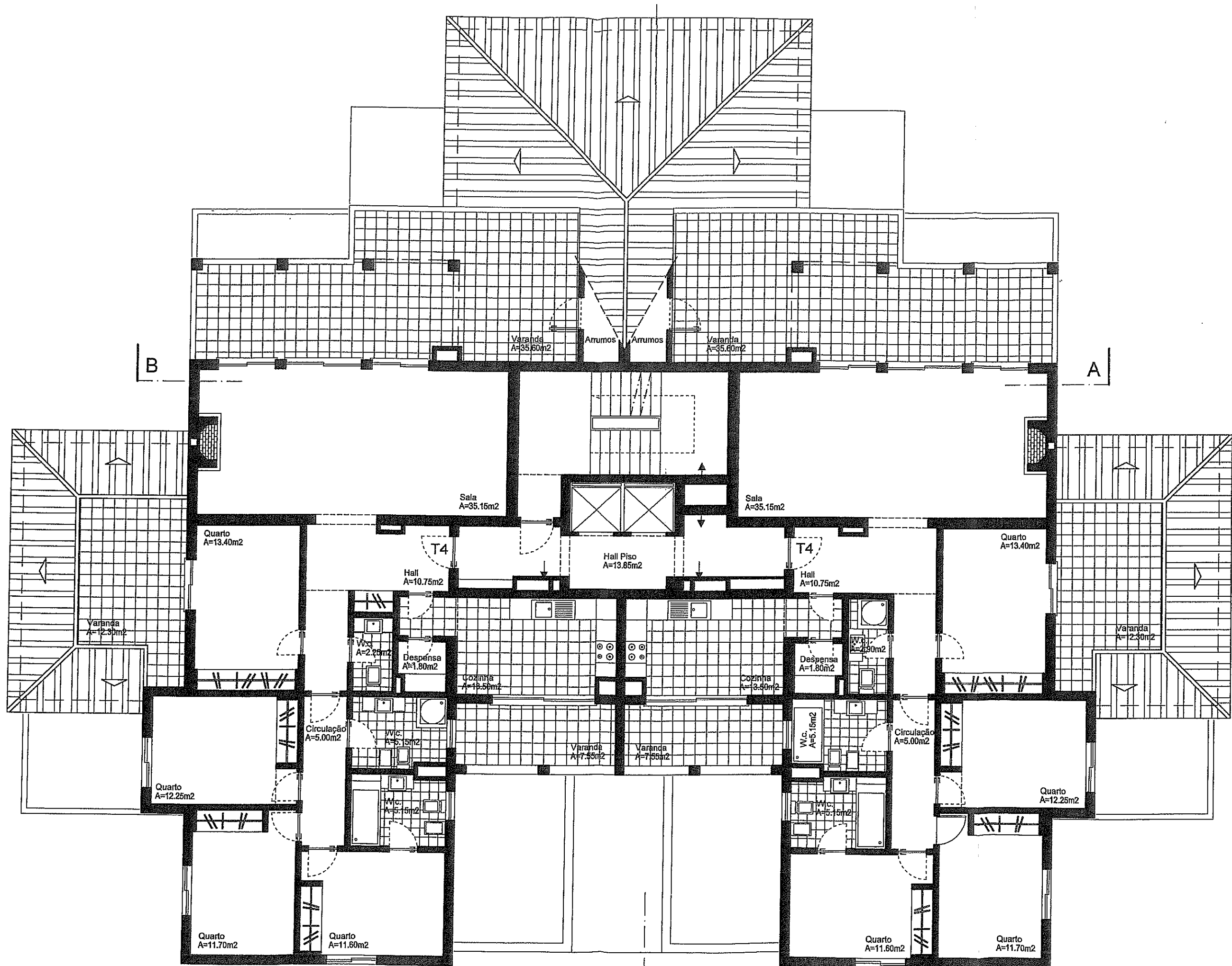
PLANTA DO PISO 4
