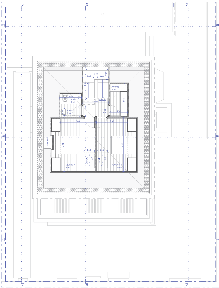
3. Planta Vão Telhado 1:100
