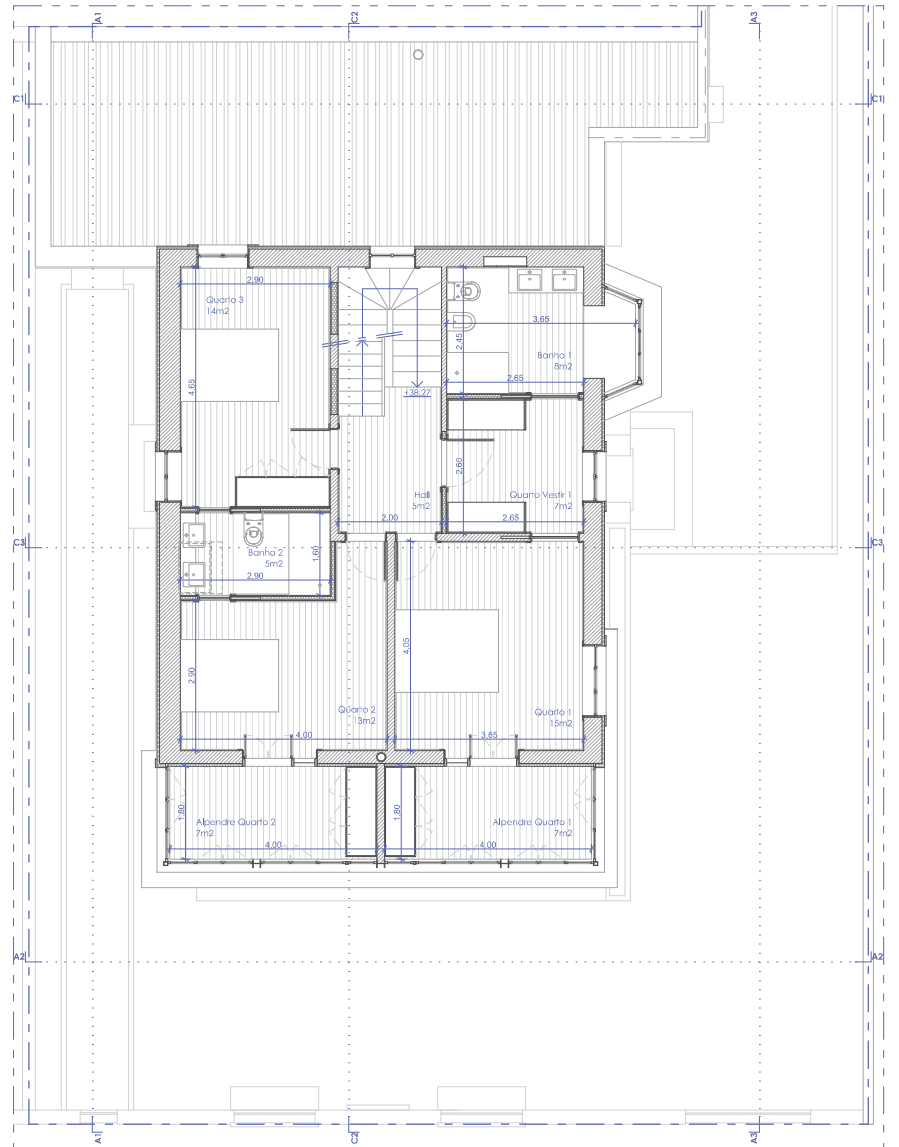
2. Planta Piso 2 - Piso Quartos 1:100
