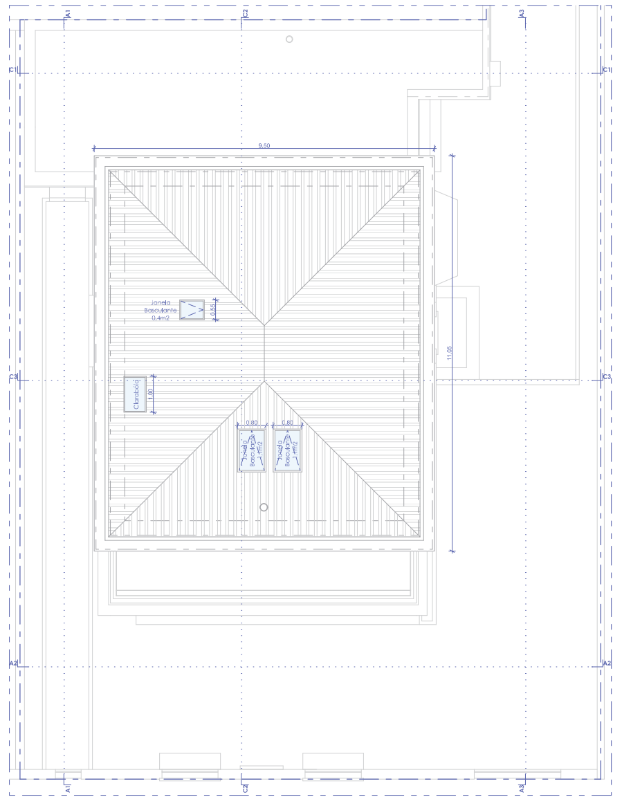
4. Planta Cobertura 1:100
