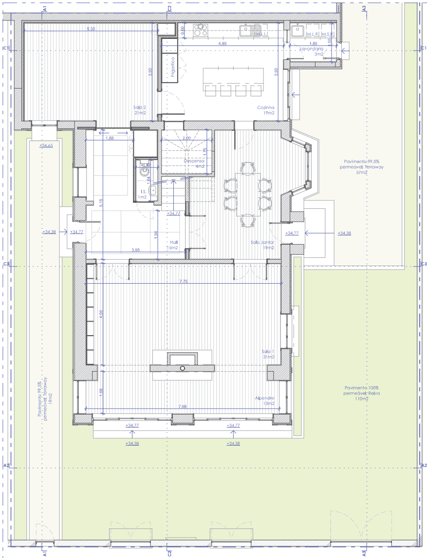
1. Planta Piso 1 - Piso Térreo 1:100
