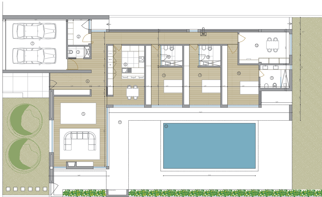
PLANTA PISO 0
