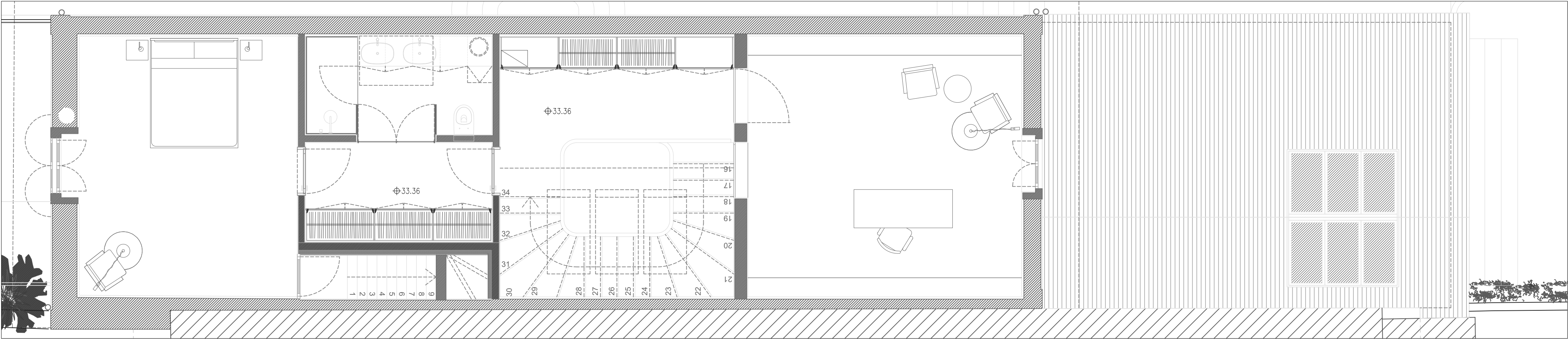
PLANTA PISO 1
