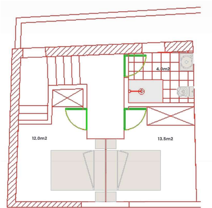
Piso 1 ABP 36,0m2
