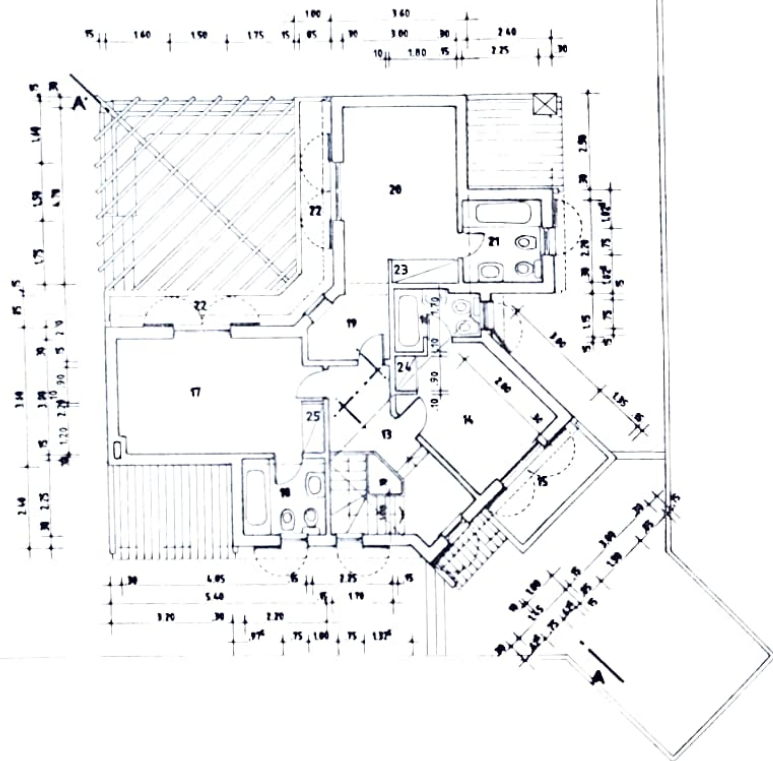
PLANTA DE 1º ANDAR
