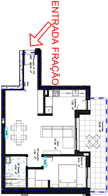
Pormenor Fração M (Piso 1)
