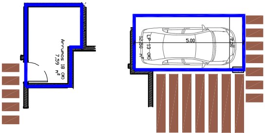
Pormenor Estacionamento/Arrumos (Piso -1)
