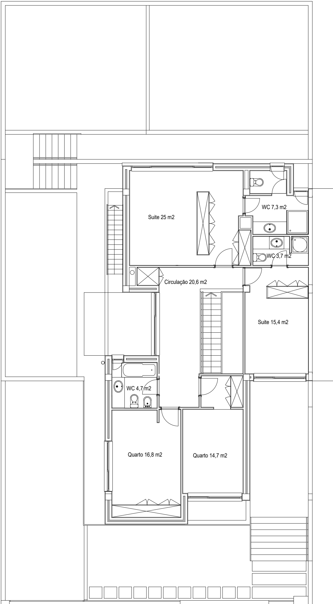
planta do 1º andar
