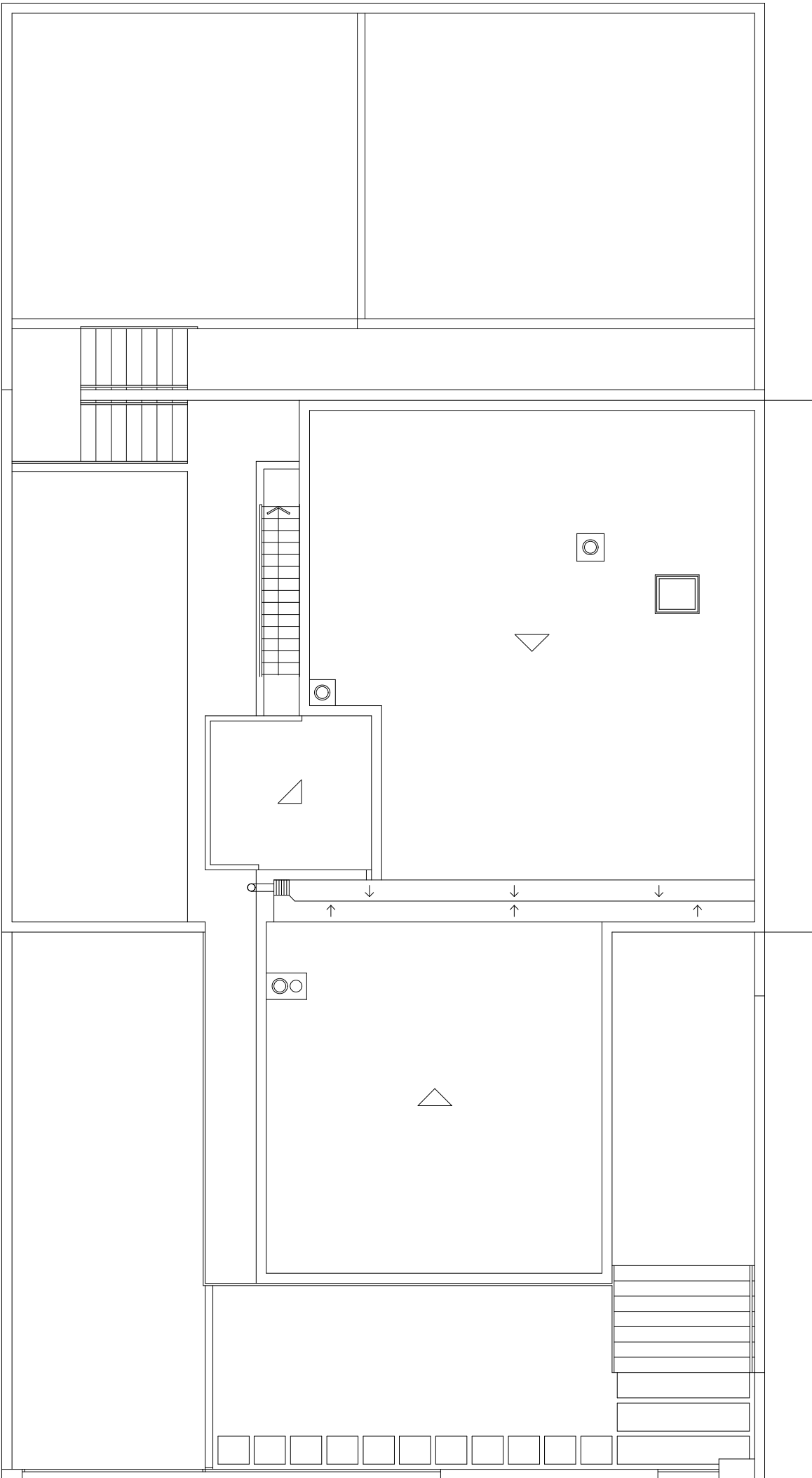
planta da cobertura
