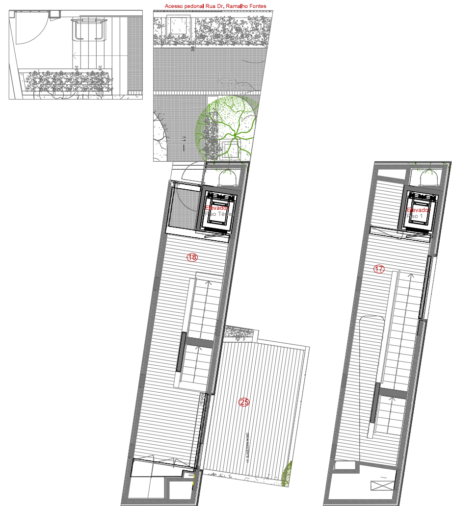
PISO TÉRREO
