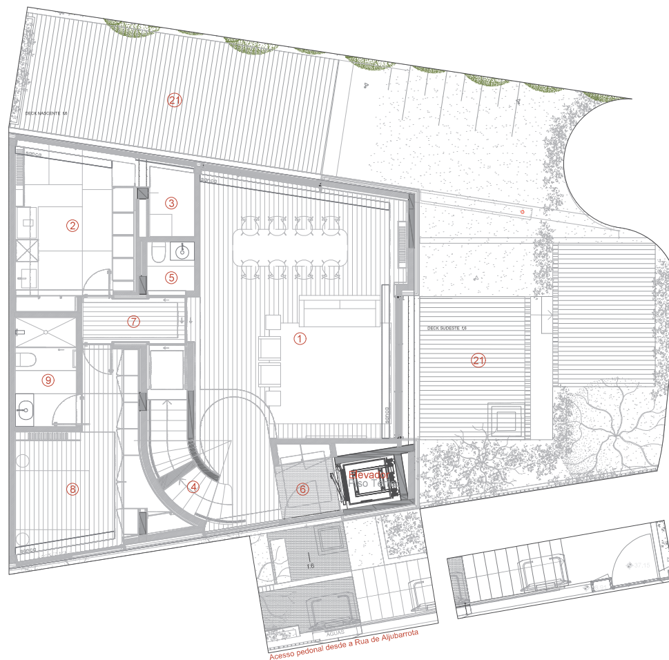
PISO TÉRREO
