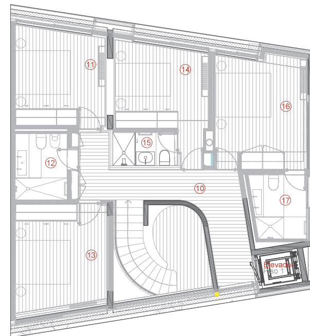
PISO 1
