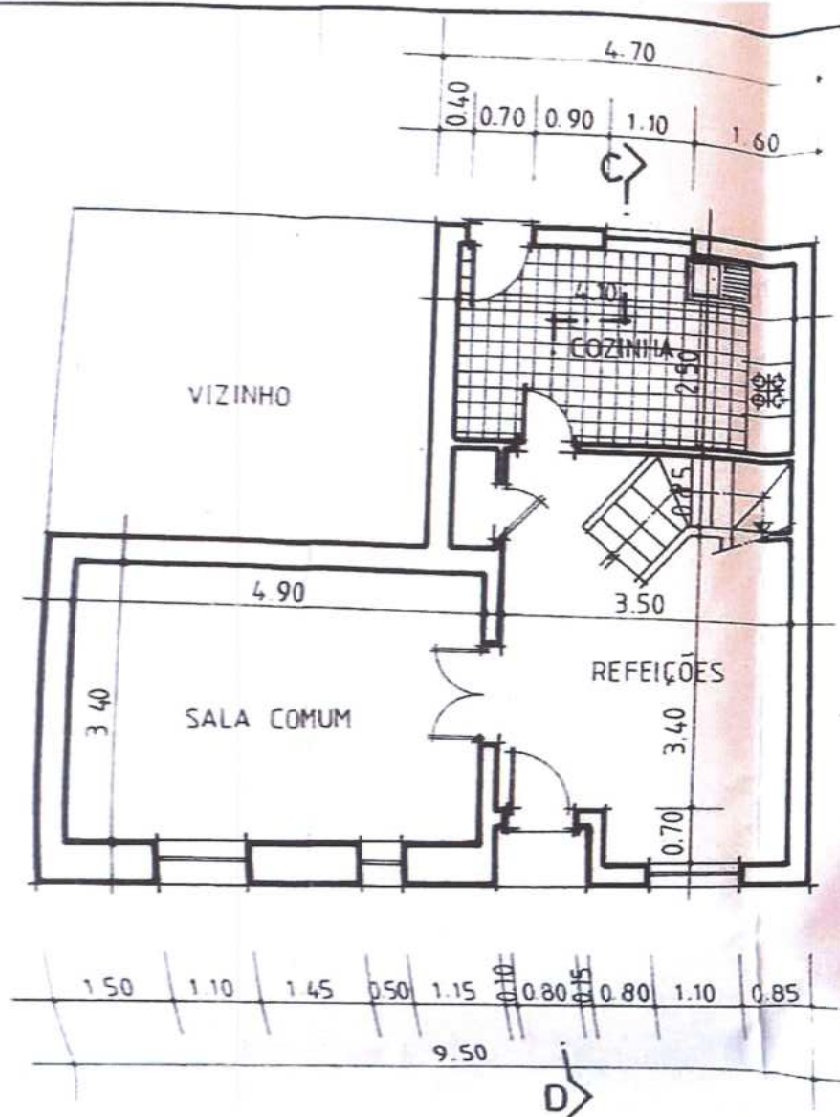
PLANTA DO R/CHÃO
