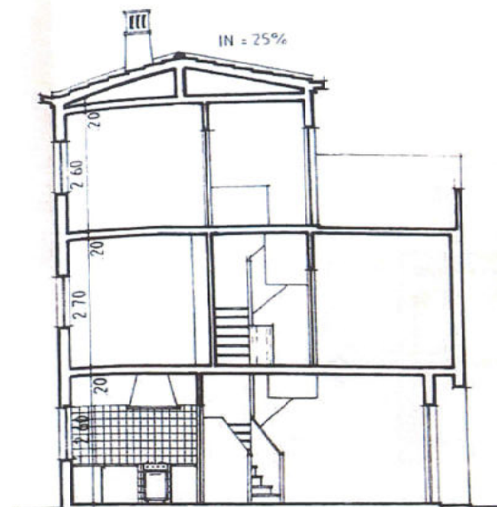
CORTE C-D
