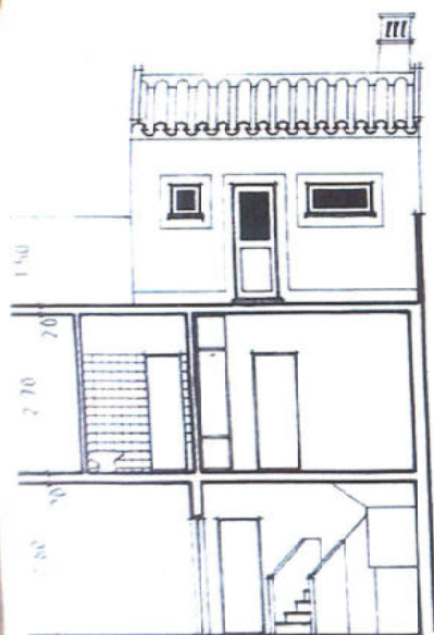
CORTE C-D
