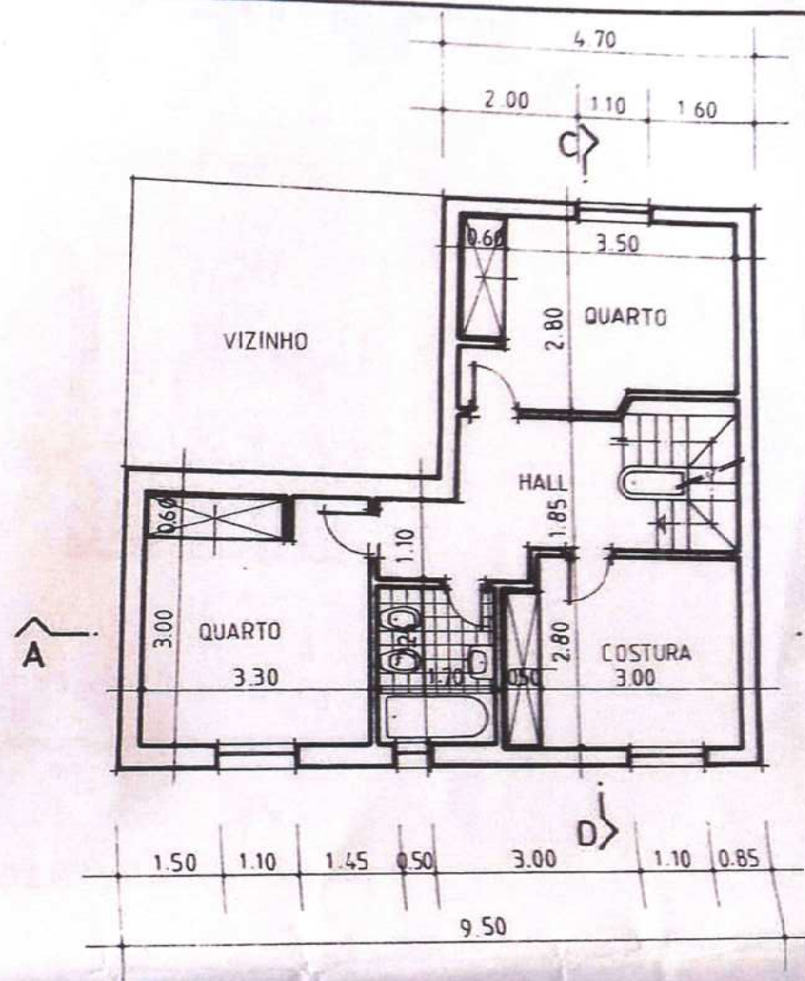
PLANTA DO 1º ANDAR
