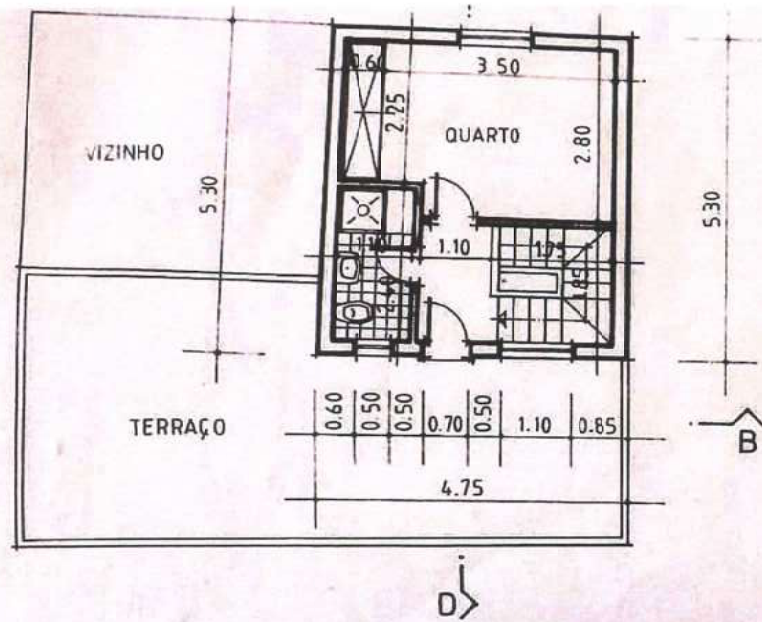
PLANTA DO 2º ANDAR
