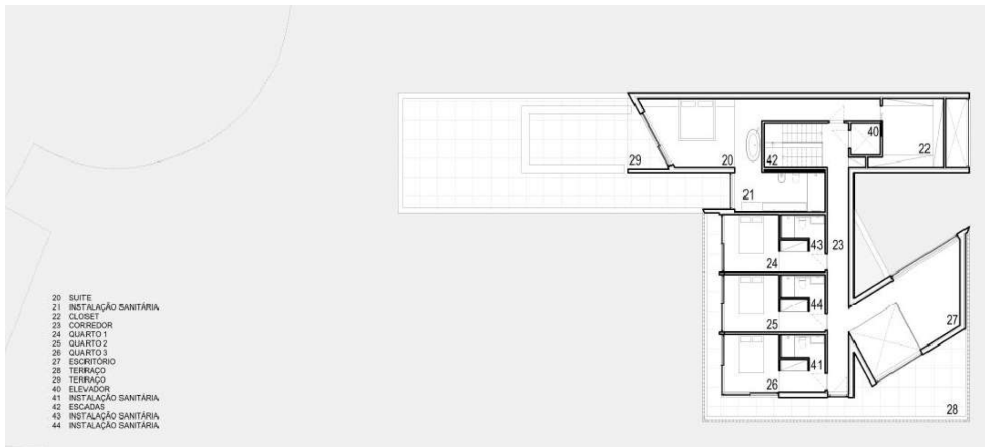
Planta Piso 1
