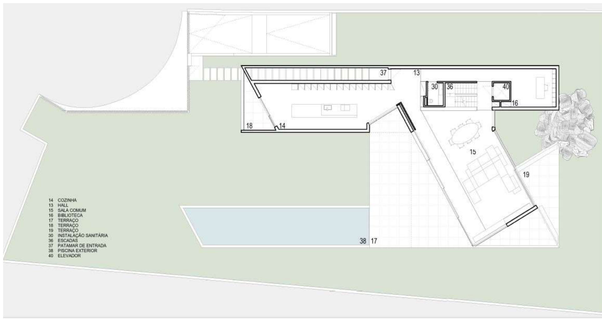
Planta Piso 0
