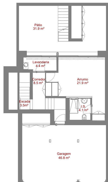
Planta Piso -1
