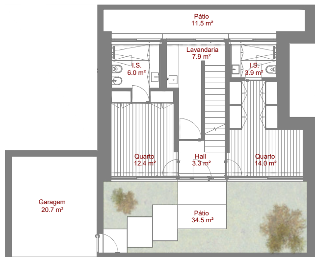
Planta Piso -1
