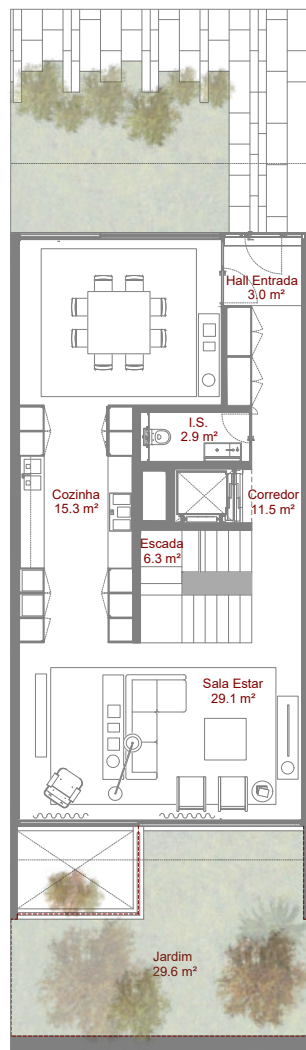
Planta Piso 0
