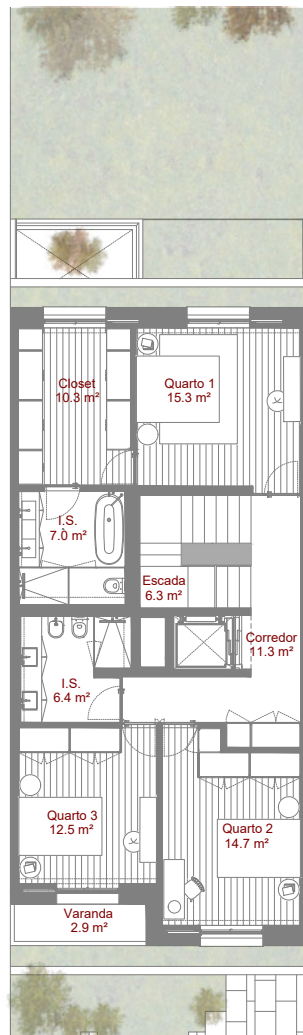
Planta Piso 1
