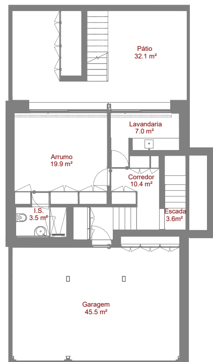
Planta Piso -1
