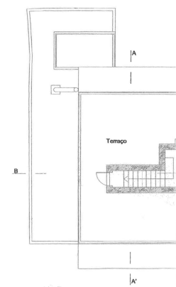
Planta do terraço
