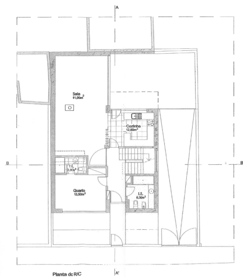
Planta do R/C
