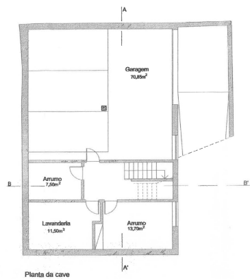
Planta da cave
