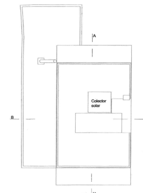
Planta do coletor solar
