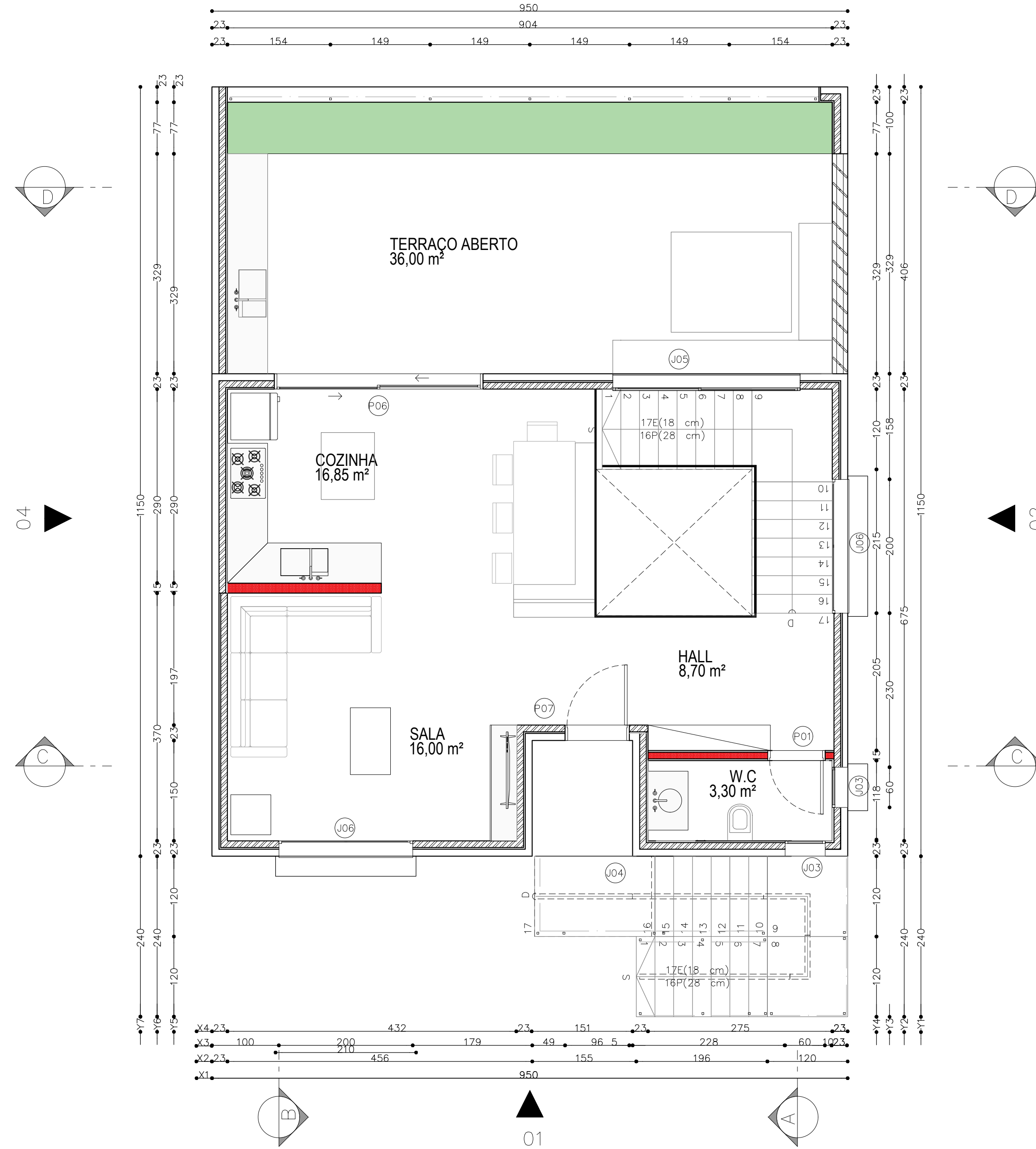
Piso 2 1:50
