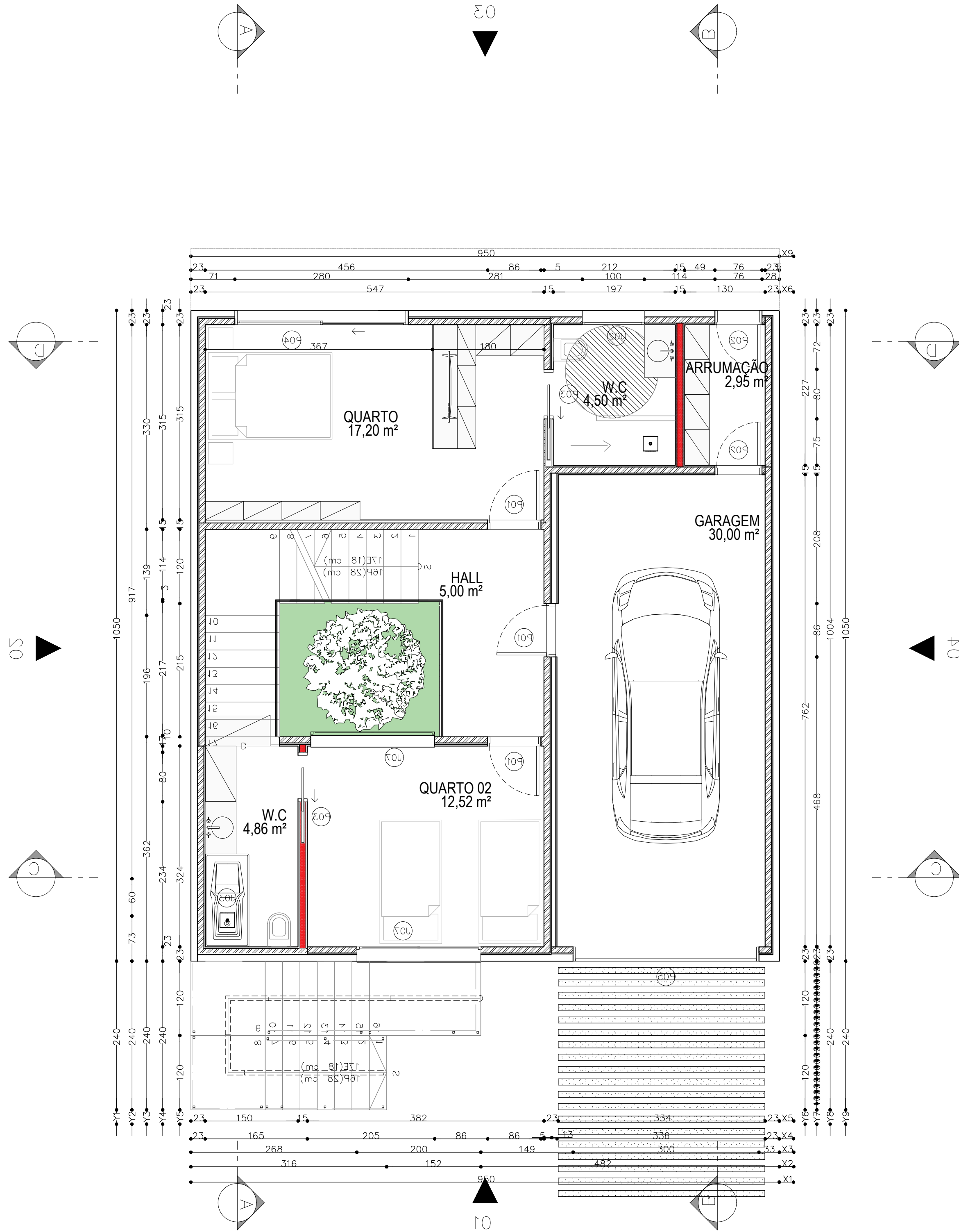
Piso 1 (R/C) 1:50
