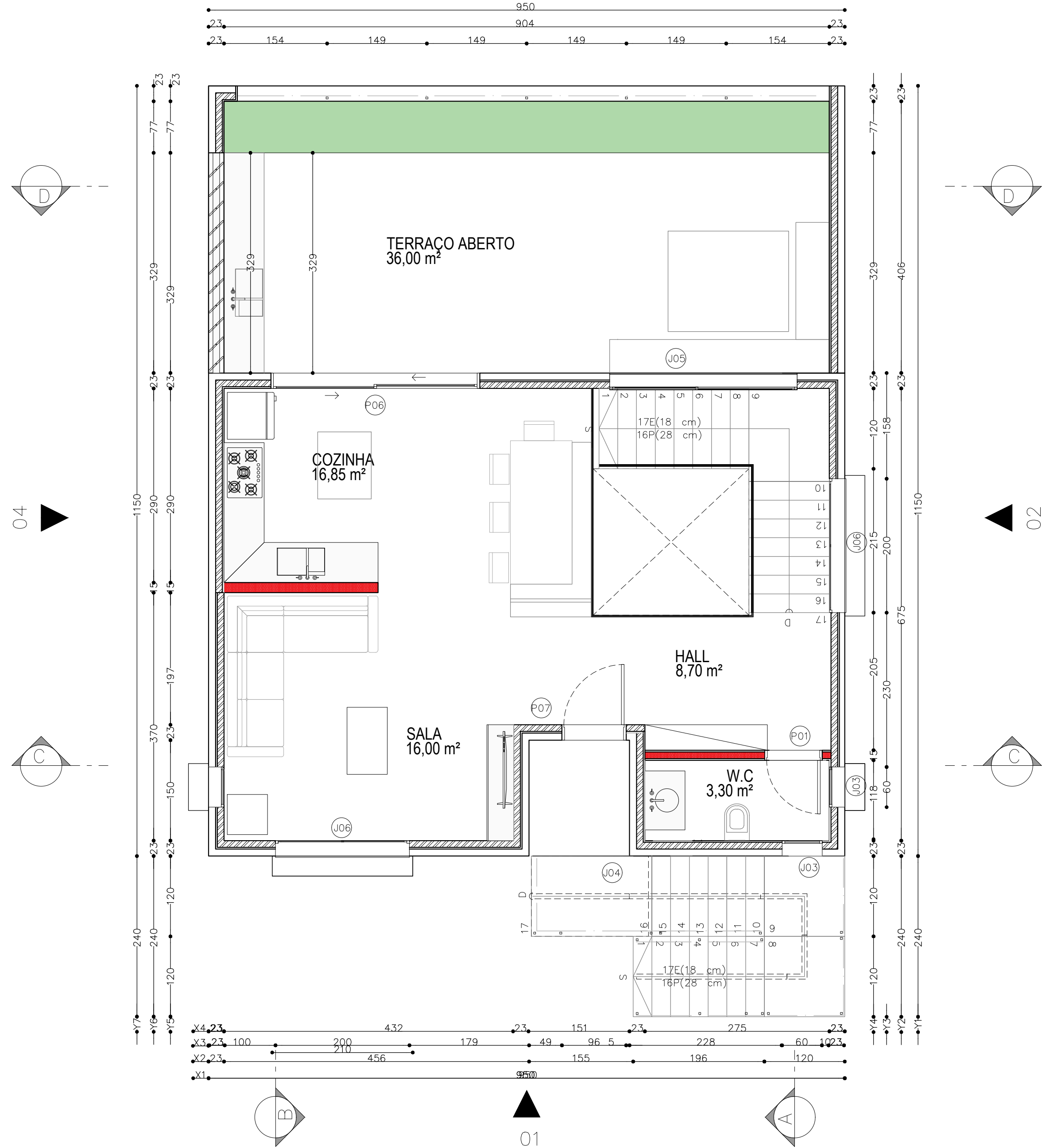
Piso 2 1:50
