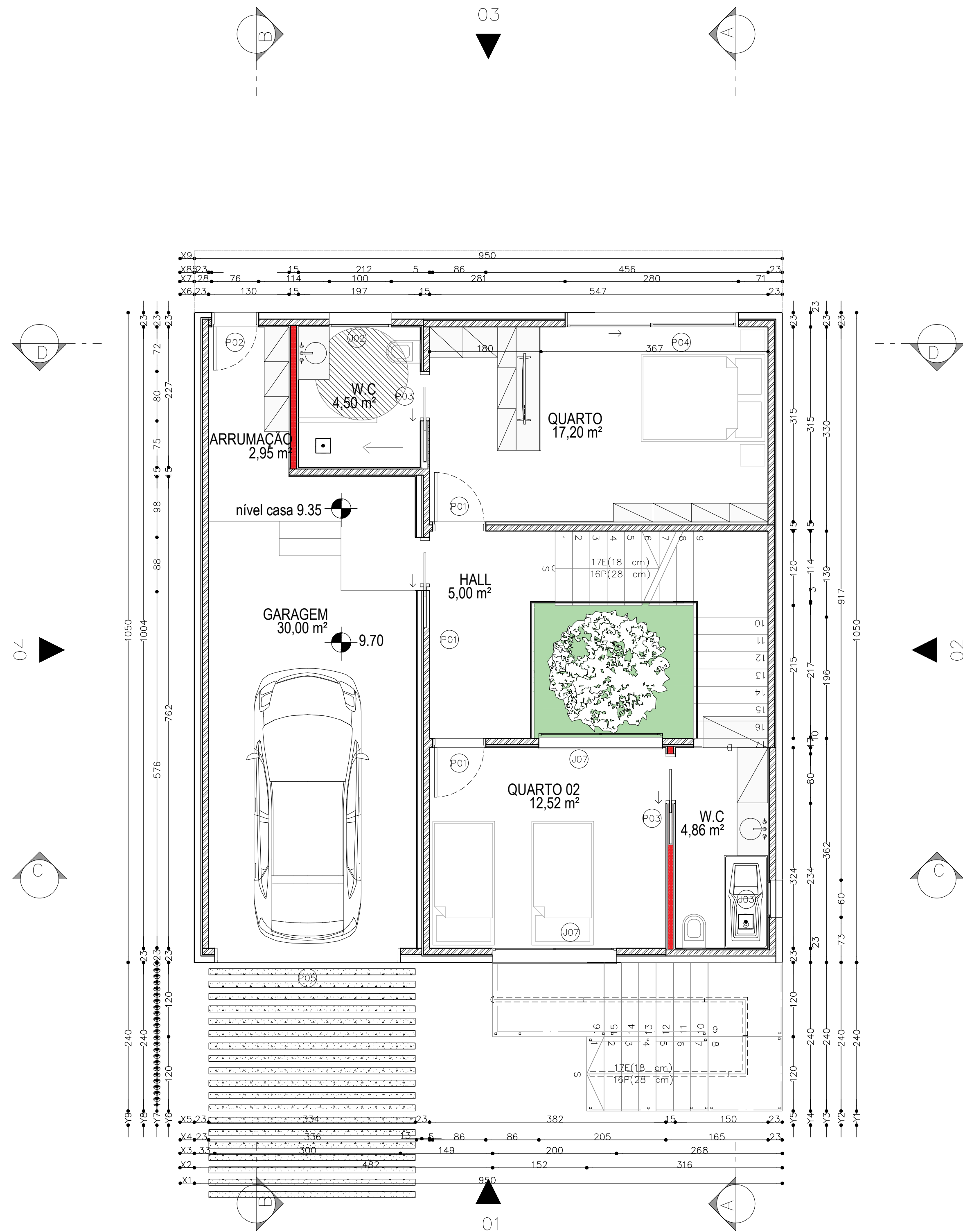
Piso 1 (R/C) 1:50
