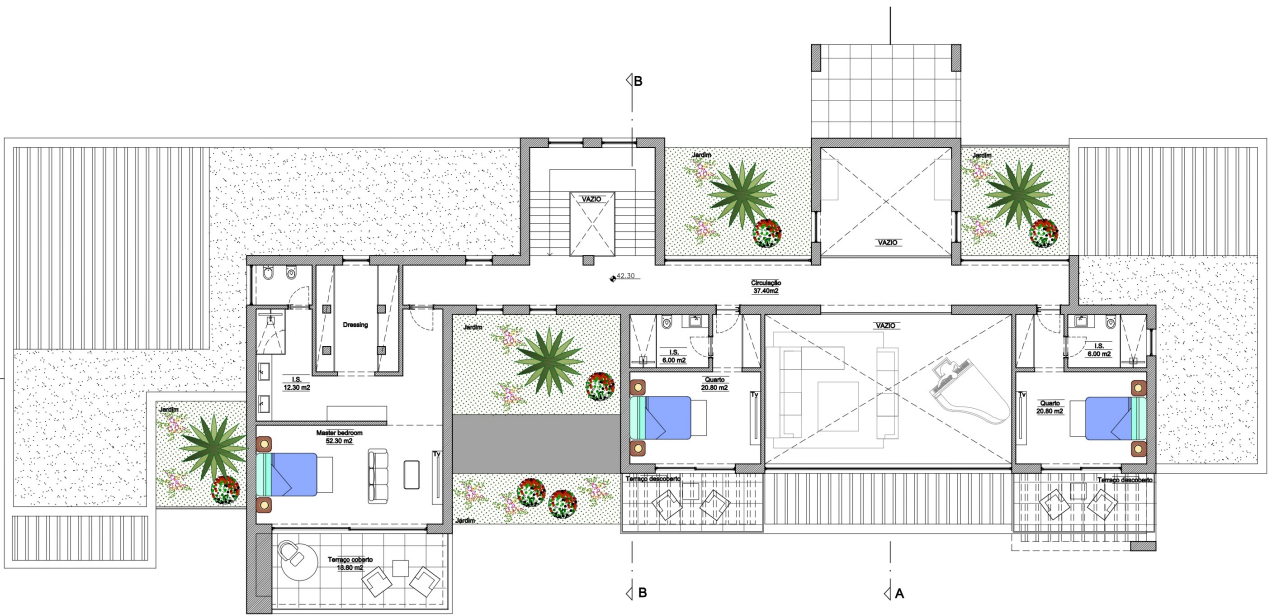
PLANTA DO 1º ANDAR - PROPOSTO
