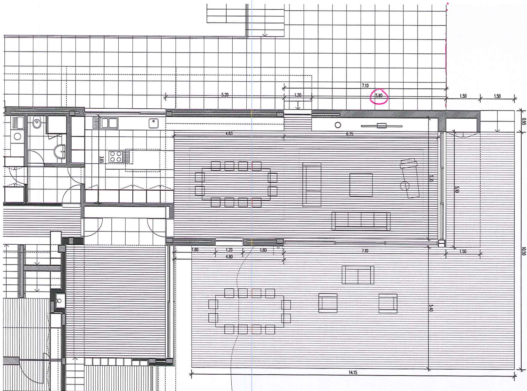
PLANTA COZINHA / SALA JANTAR E ESTAR - versão 1
