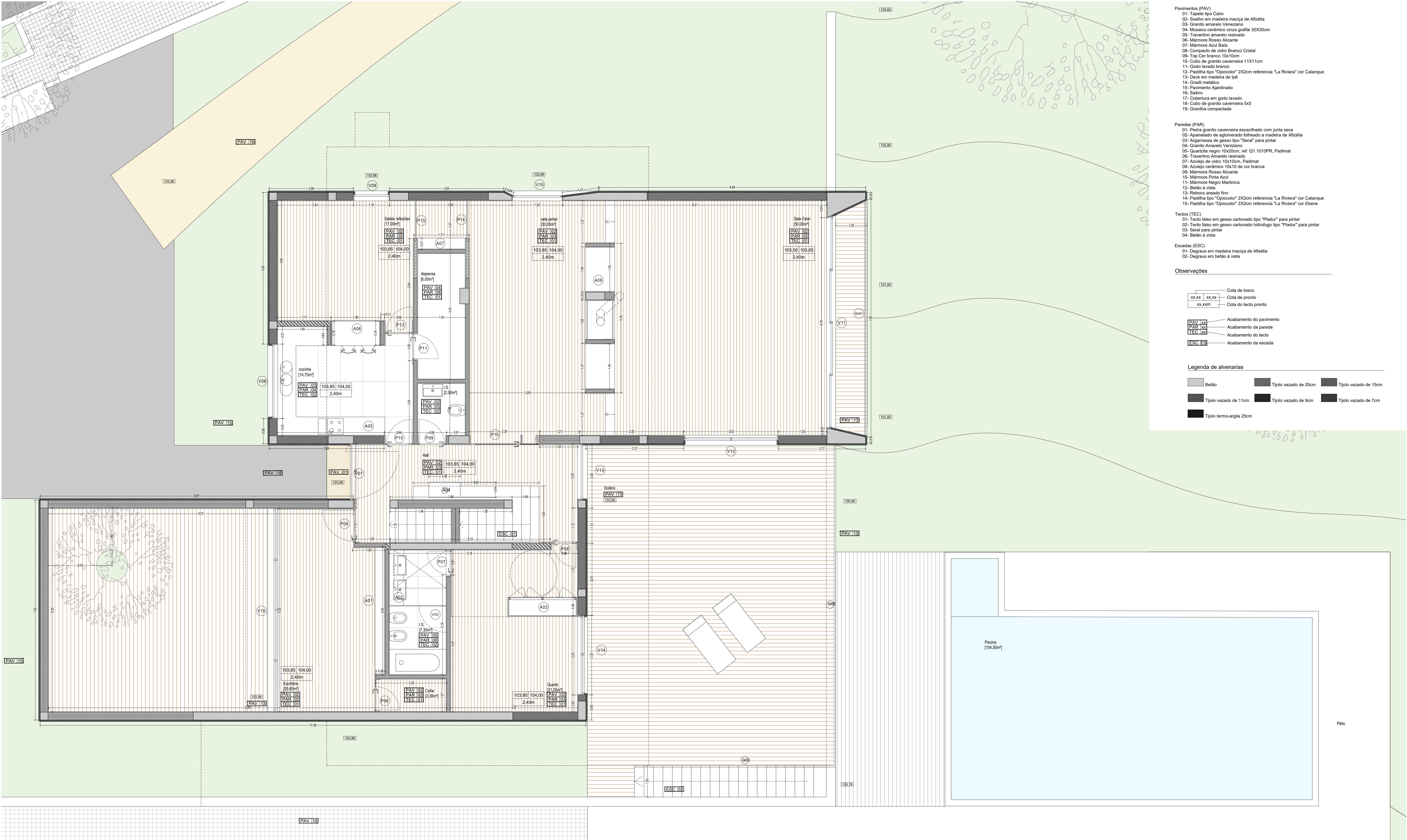
Planta de R/Ch - escala 1:50
