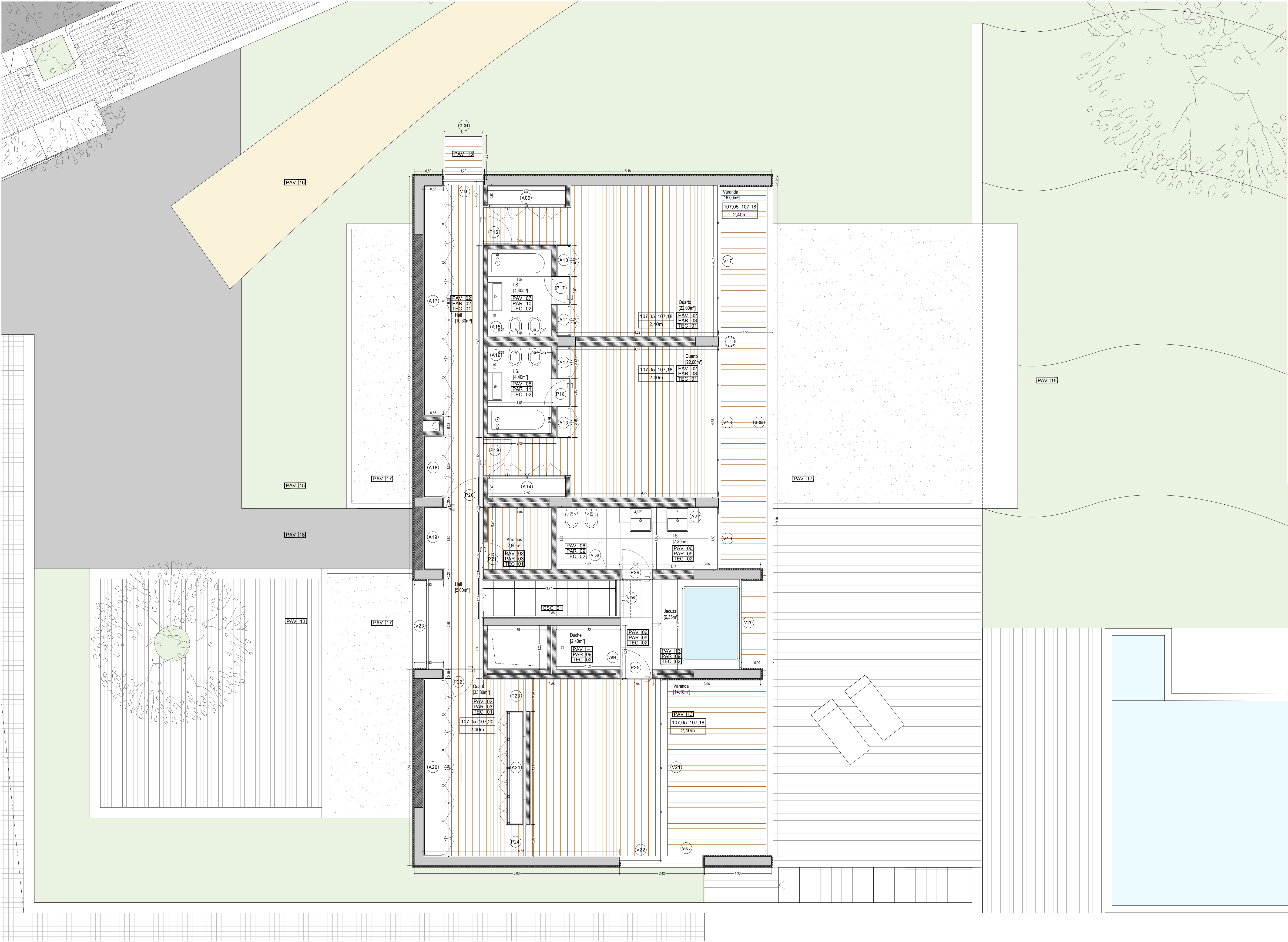
Planta de 1º Piso - escala 1:50
