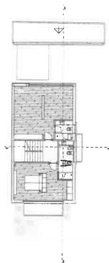
PLANTA DO 2º ANDAR
