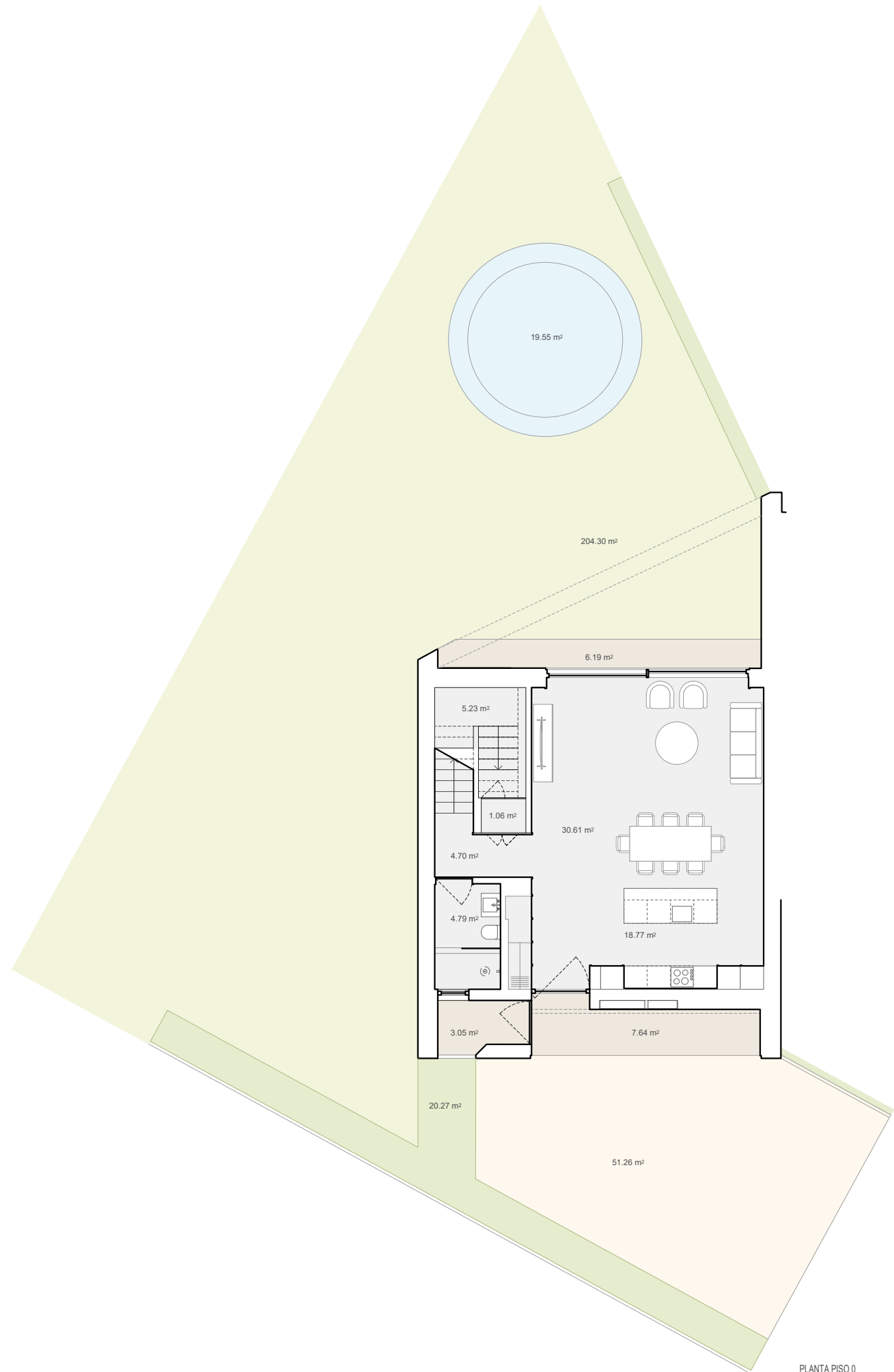
PLANTA PISO 0
