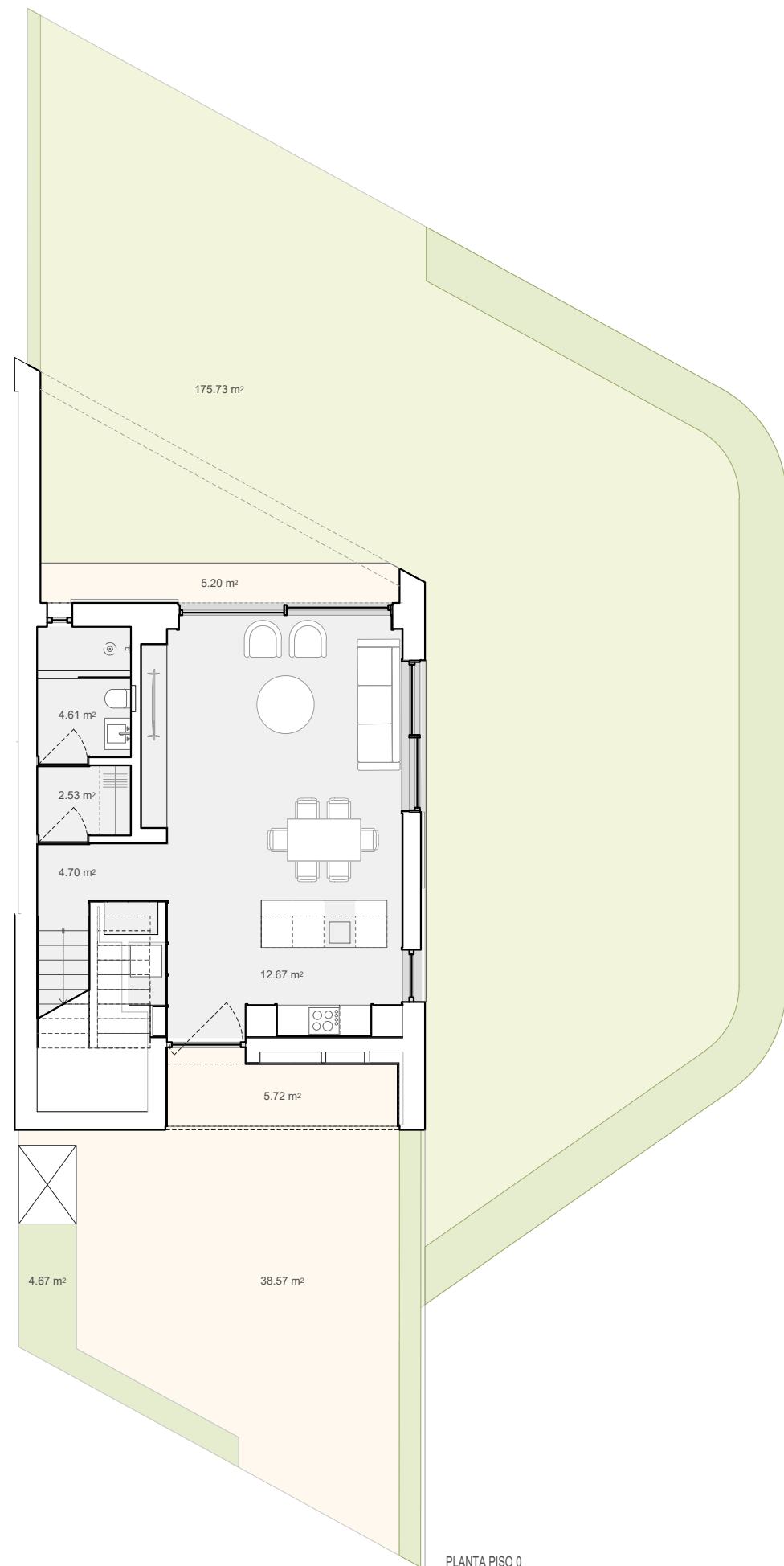
PLANTA PISO 0
