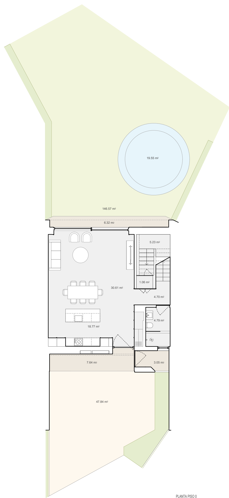
PLANTA PISO 0
