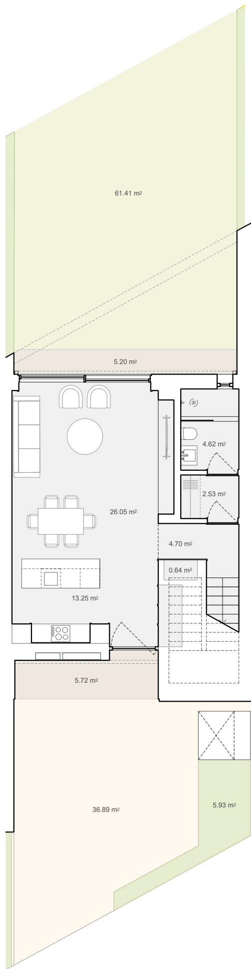
PLANTA PISO 0
