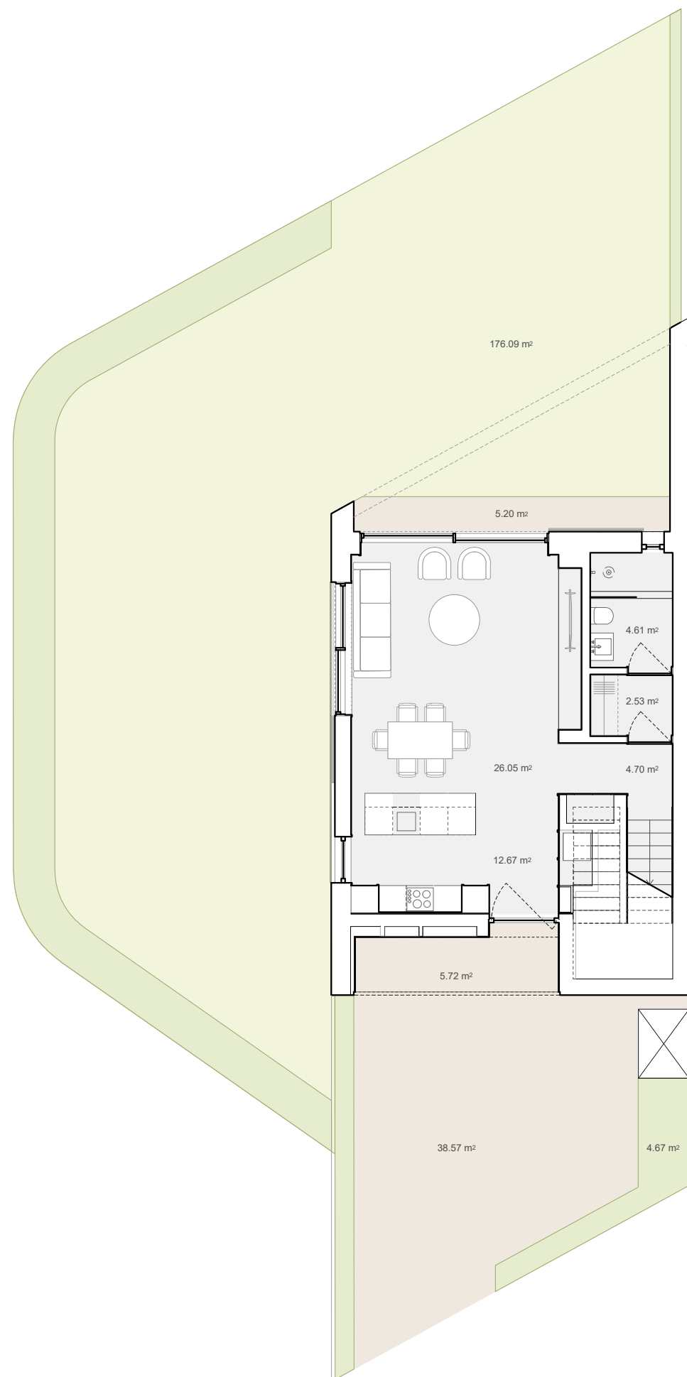
PLANTA PISO 0
