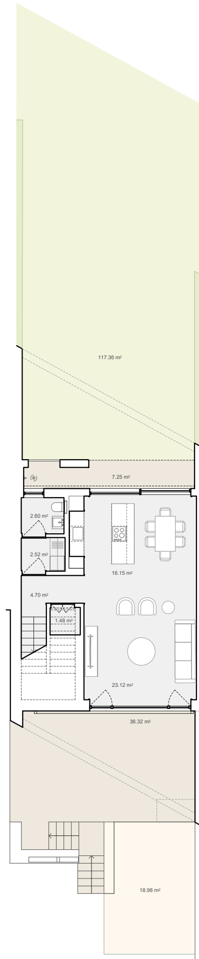
PLANTA PISO 0
