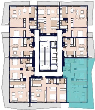
SEGUNDO ANDAR
